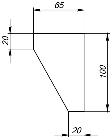
Поз.2 (Ребро)
